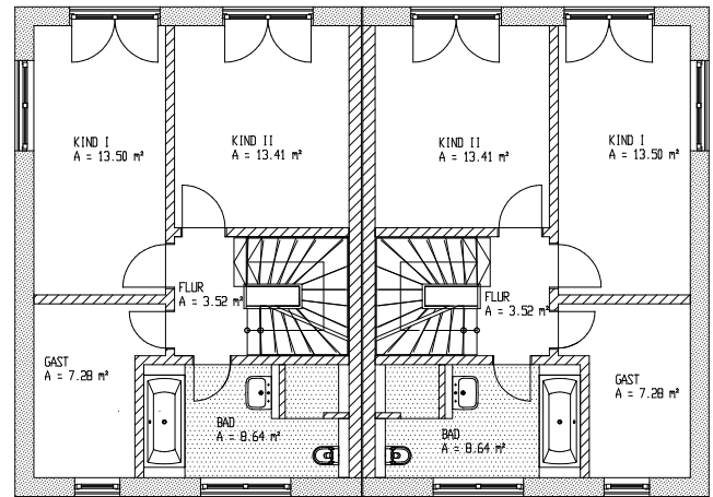
Obergeschoss: Wohnnutzfläche ca. 47 m 2
