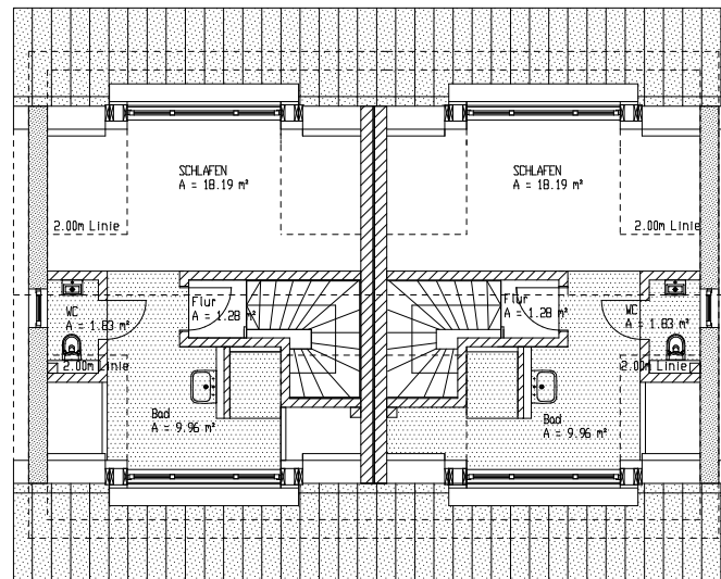
Obergeschoss: Wohnnutzfläche ca. 47 m 2
