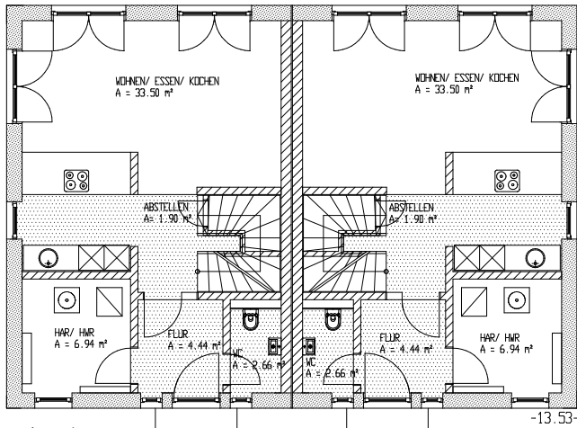
Erdgeschoss: Wohnnutzfläche ca. 50 m 2
